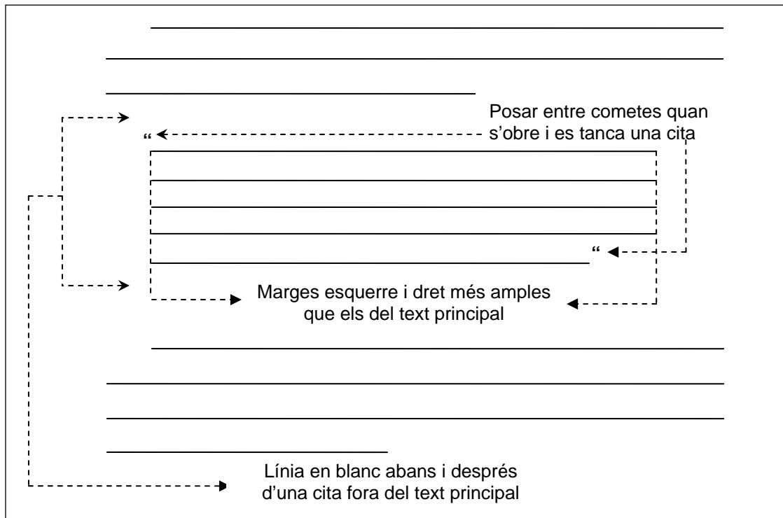
Figura 1.6.: Citacions textuals
